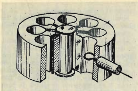
Sopra: Sezione di un «magnetron» a più cavità. Si noti il catodo, l'anodo con otto cavità, la sonda per raccogliere l'energia R.F.
