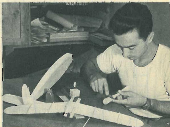
Incollatura del dorso della fusoliera.
