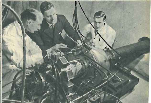
Sopra a destra: La turbina al banco di prova. Il complesso è costituito da un compressore, due camere di combustione, ed una turbina collegata alle ruote tramite un riduttore. Compressore e turbina non sono collegati meccanicamente. Sotto: la vettura sperimentale è a motore posteriore.
